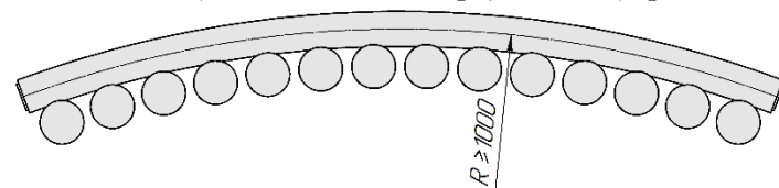
Гармония А 40-1 R наружн. (вид сверху)
