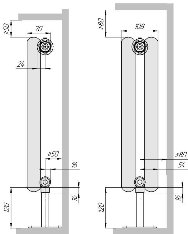
Гармония С40 1 нп нв (вид сбоку)
