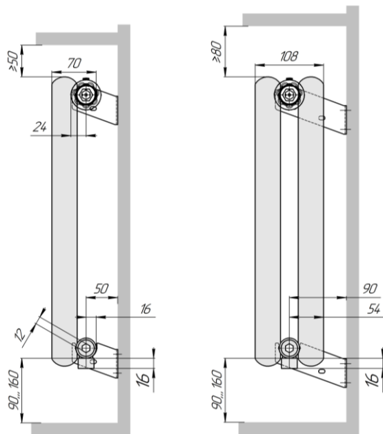
Гармония С40 1 нп (вид сбоку, кронштейны С 50) Гармония С40 2 нп (вид сбоку, кронштейны С 90)
