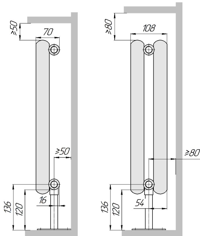
Гармония С40 1 нв (вид сбоку)
