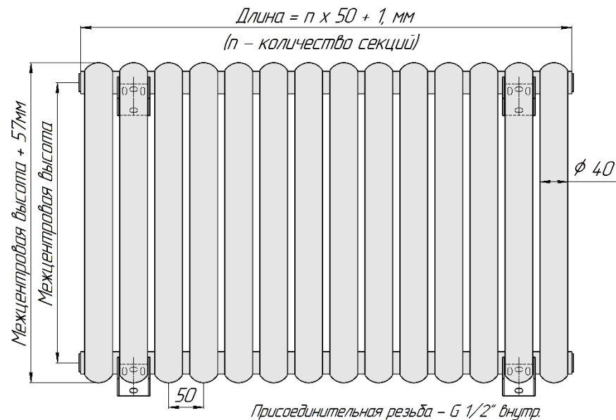
Гармония А40 1 (вид сверху)
