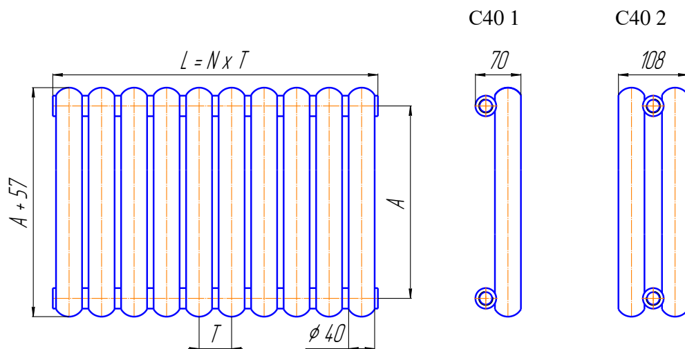
Рис. 1 Радиатор «Гармония С40», где: А – межцентровый размер, мм; Т – шаг (Т = 50 мм); N – количество секций; L – габаритная длина, мм.
